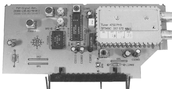
Signal Modul mit Splitter Signal Module with Splitter
