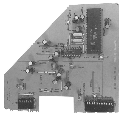
PIP-Baustein / PIP Module
